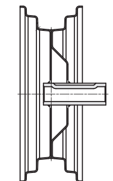
TUBO CILINDRICO SEDE CHIAVETTA KEY SEAT PIPE
